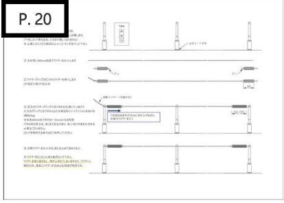
A rod UBS-T0 Φ1.2 UBW roll + UBW-Grip
