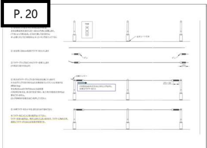
B rod UBS-T0, T0-B, T0 DD Φ0.8 UBWM roll + UBWM-Grip
