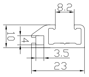
UIA-PR<ロール>断面図
